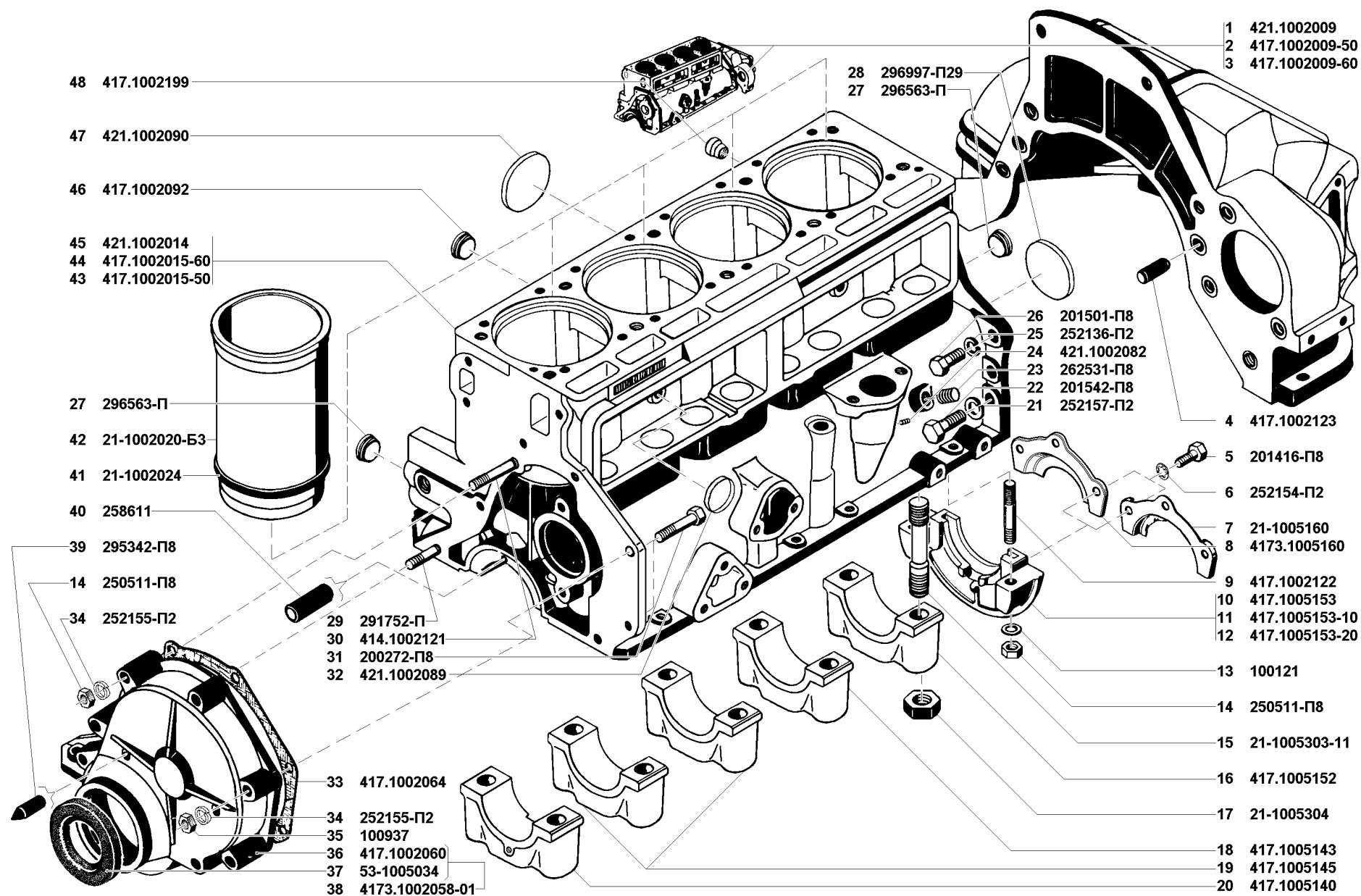
Рис. 3. Блок цилиндров (1002)
